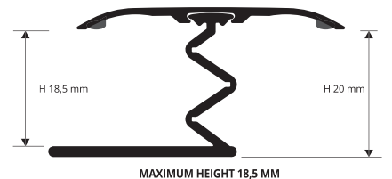
PMPFX... 42090AS / 42A + PMFIXBSAN 23 scale 1:1
